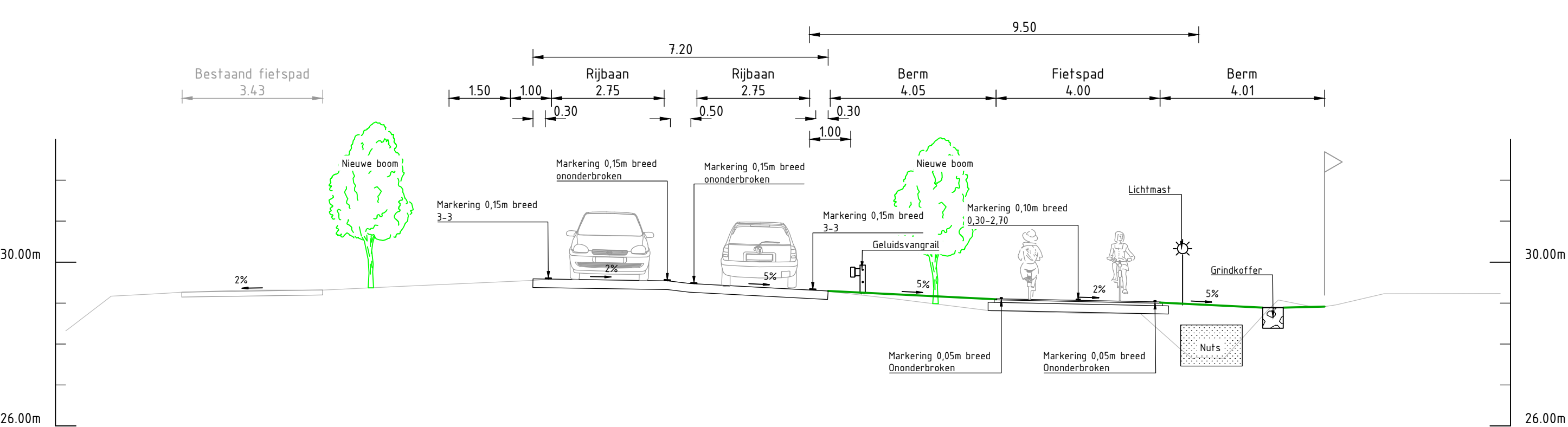
Dwarsprofiel DWP-61 Schaal 1:100
