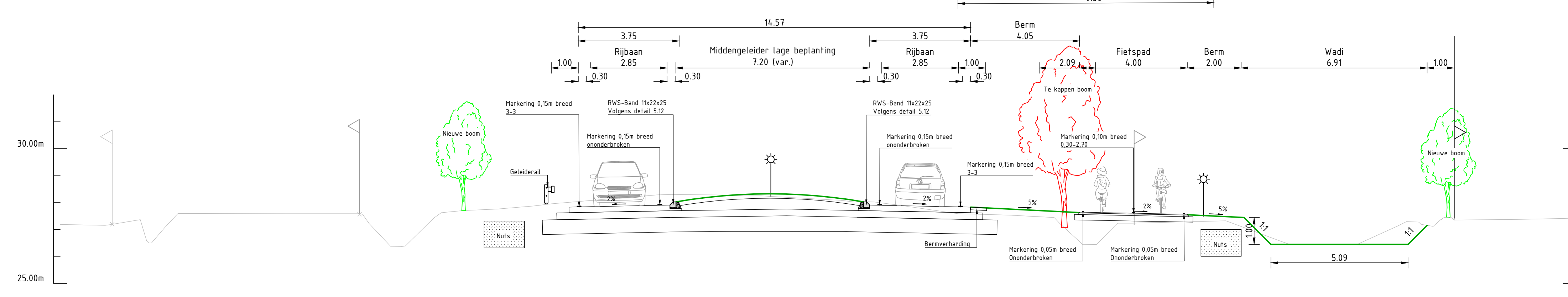
Dwarsprofiel DWP-54 Schaal 1:100
