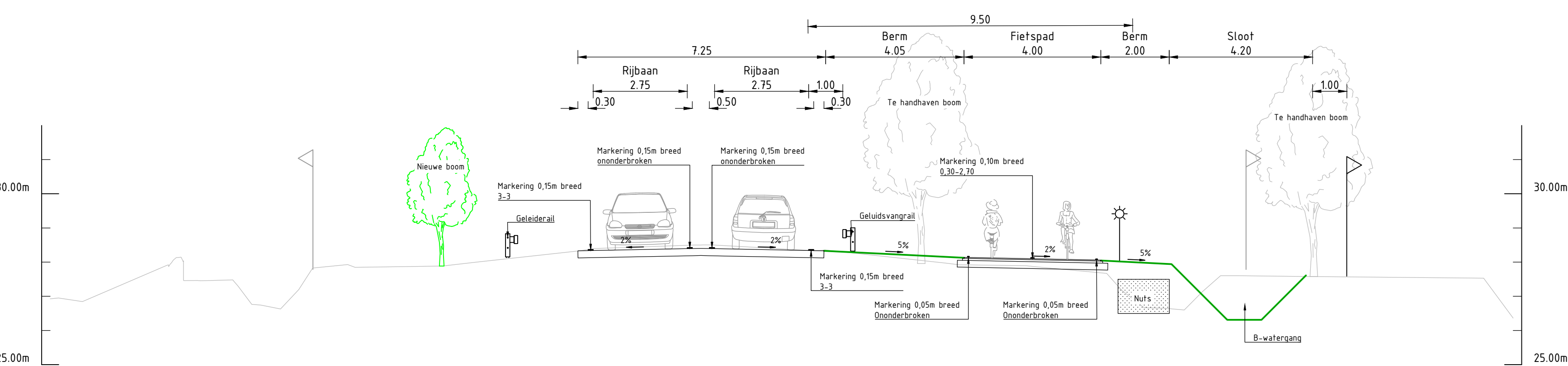
Dwarsprofiel DWP-55 Schaal 1:100
