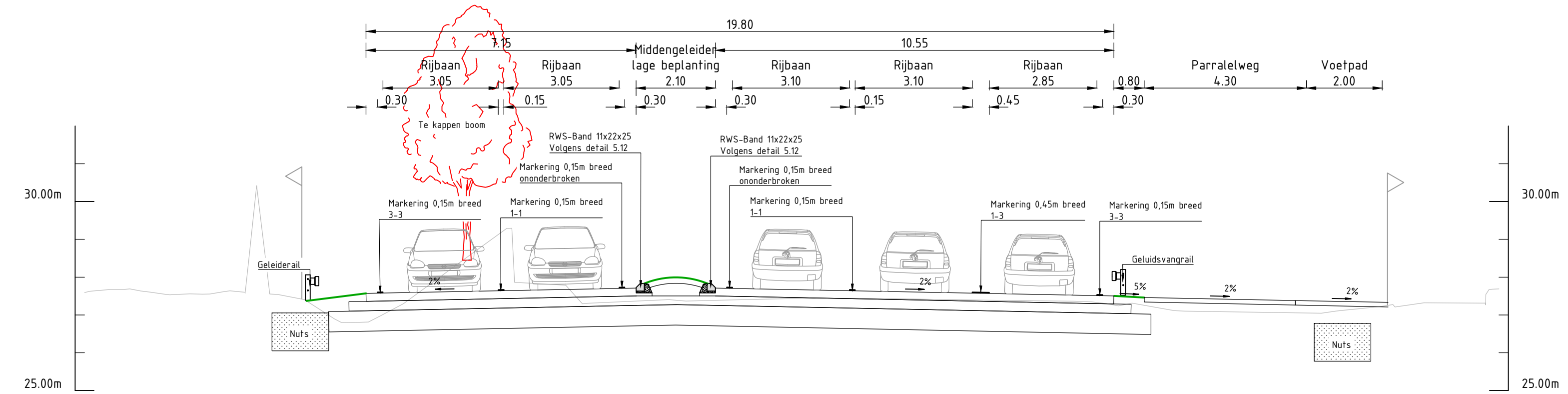
Dwarsprofiel DWP-52 Schaal 1:100
