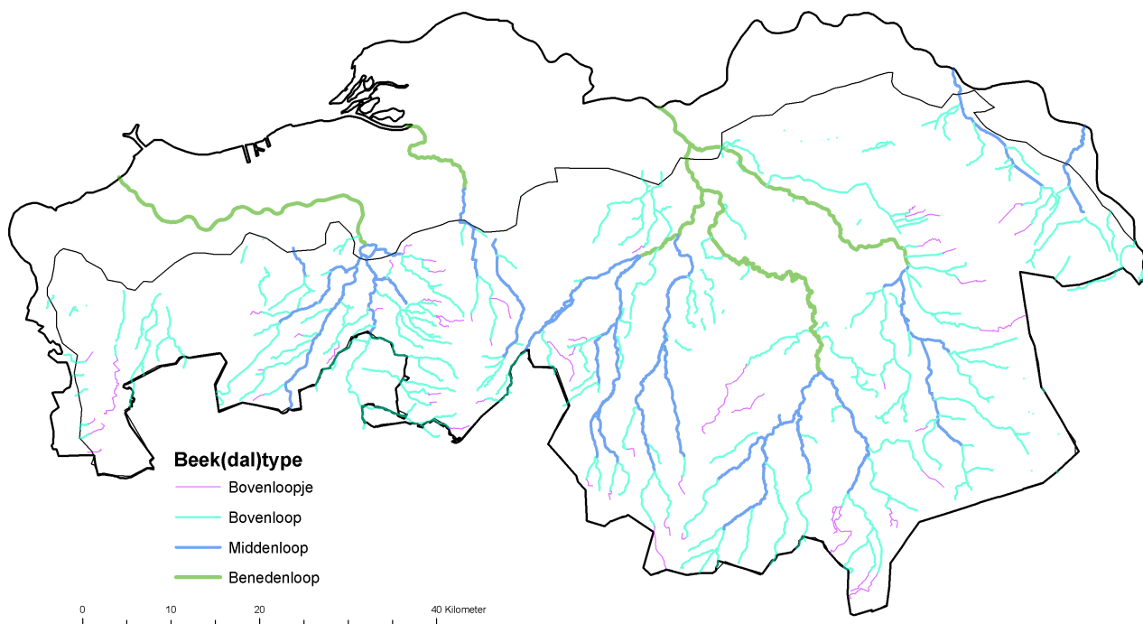
Figuur 2-4 Indeling beeklopen naar beektype
