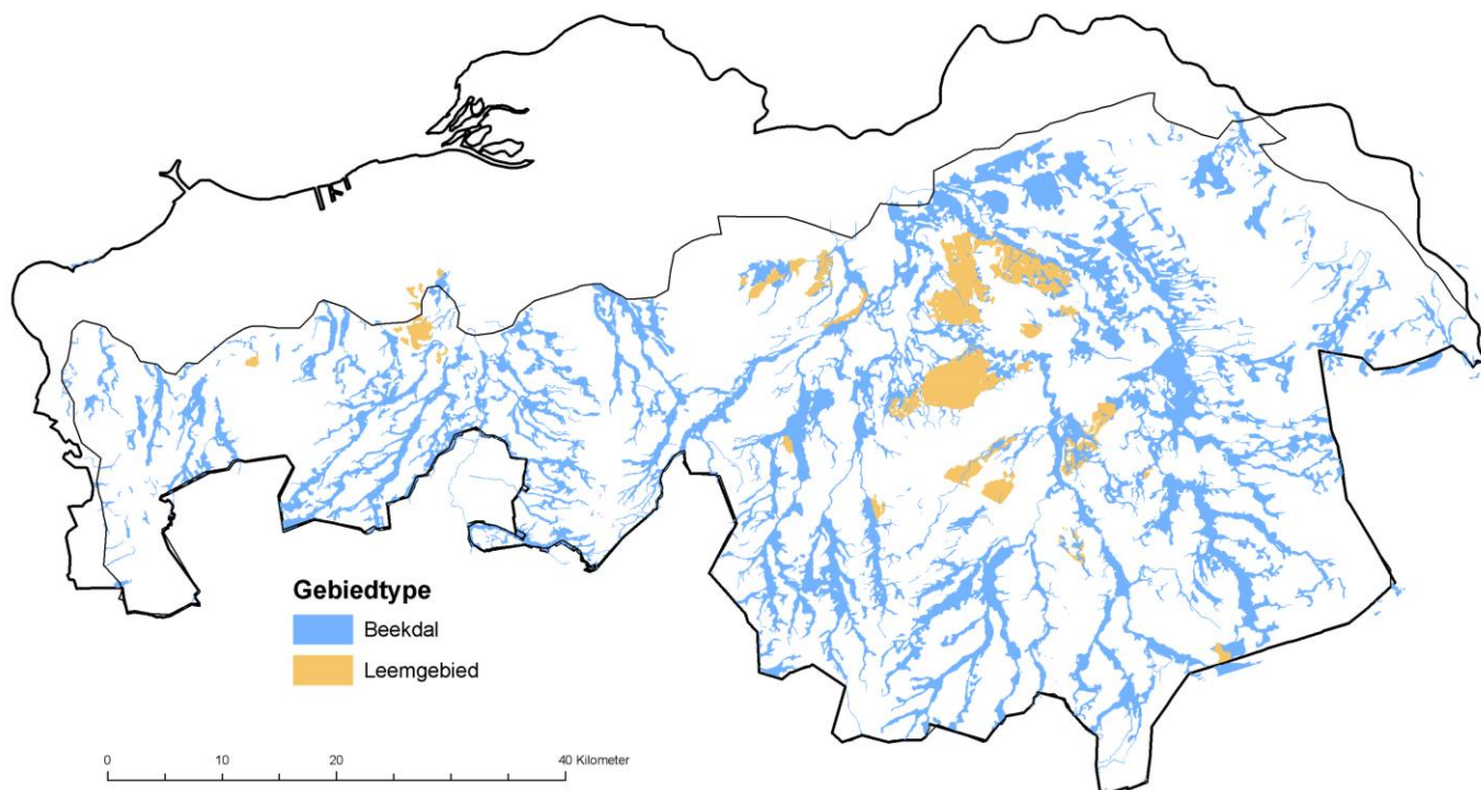
Figuur 2-2 Overzicht ligging beekdalen en leemgebieden. Dunne zwarte lijn geeft globale ligging zandgebied.
