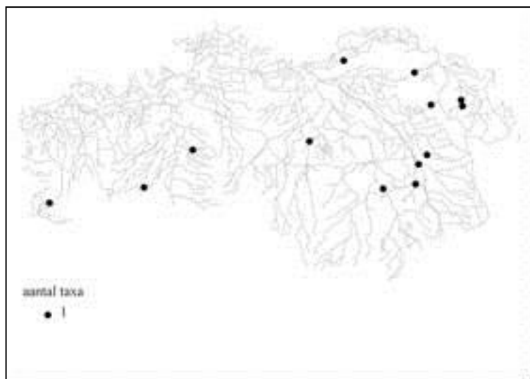
Figuur 5-10 Verspreiding soorten van zwak zure middenlopen (SG7c)
