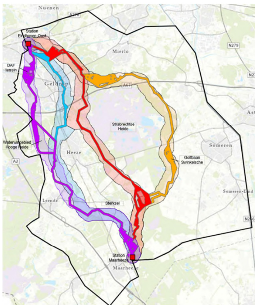
Figuur 1 Zoekgebied (zwart omkaderd) met daarbinnen de vier corridors en de alternatieven die in het MER worden onderzocht (bron: NRD).
