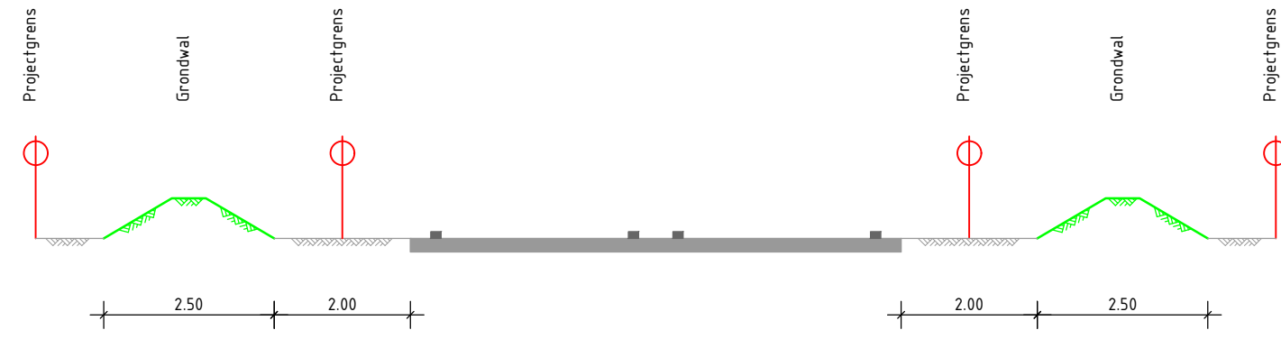
Principe dwarsprofiel L-L N285 - wegprofiel: bestaande rijbaan met grondwal Schaal 1:100
