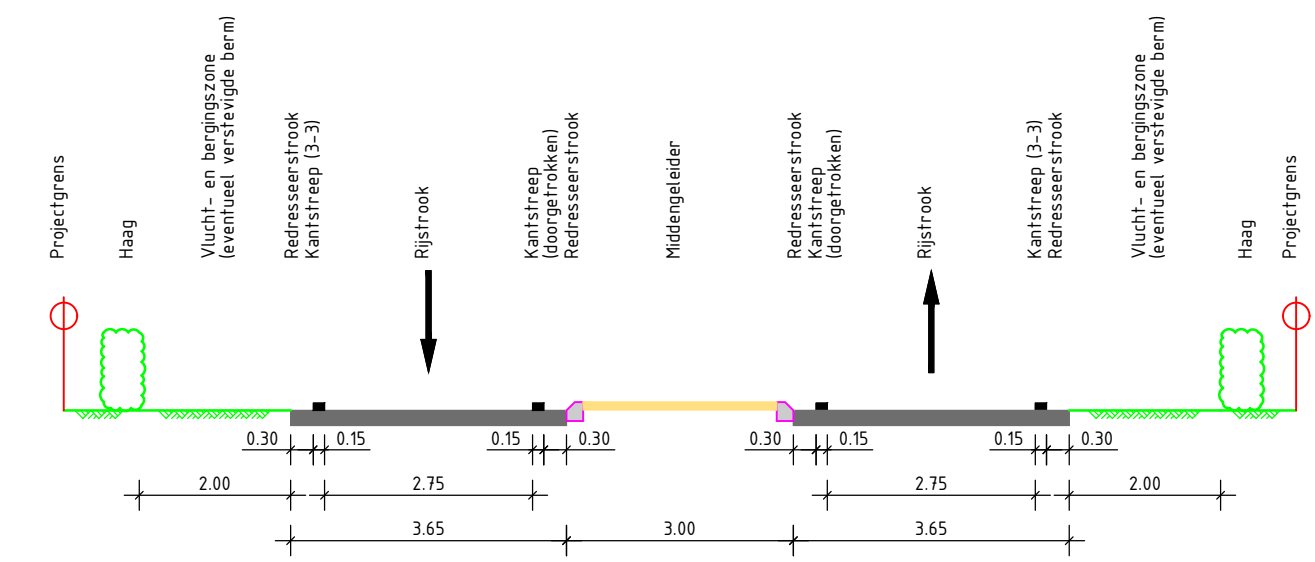
Principe dwarsprofiel D-D N285 - wegweg: rijbaan met middengleider Schaal 1:100
