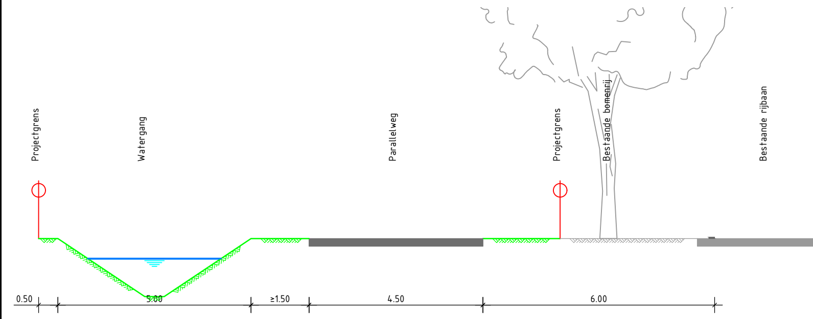
Principe dwarsprofiel E-E N285 - wegw profiel: parallelweg Schaal 1:100
