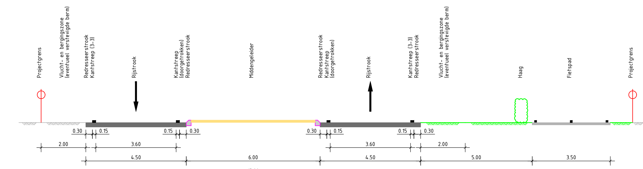
Principe dwarsprofiel F-F N285 - wegprofiel: rijbaan met brede middengeleider Schaal 1:100
