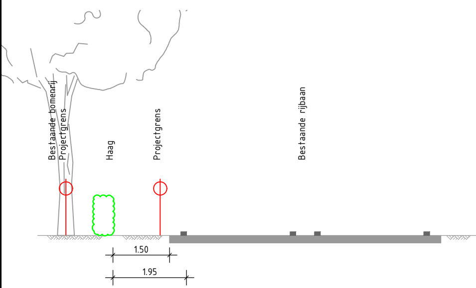
Principe dwarsprofiel K-K N285 - wegweg: bestaande rijbaan met haag Schaal 1:100
