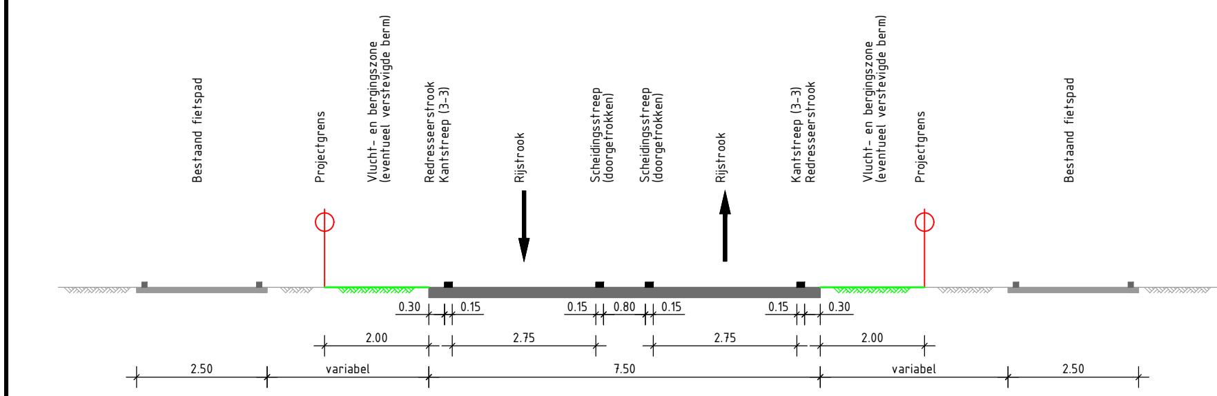
Principe dwarsprofiel A-A N285 - wegprofiel: rijbaan Schaal 1:100
