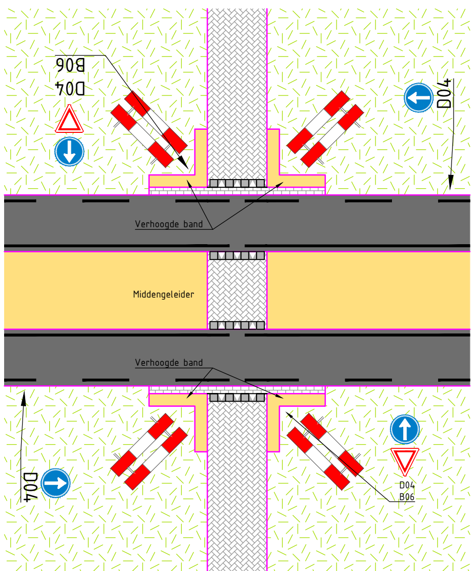
Principe inrichting koude oversteeek SCHAAL 1: 250
