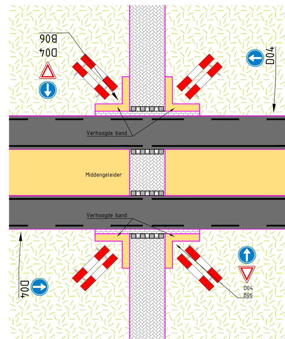
Principe inrichting koude oversteek SCHAAL 1: 250
