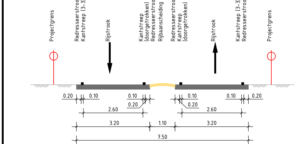
Principe dwarsprofiel H-H N285 - wegw profiel: rijbaan (60 km/h) met fysieke rijbaanscheiding Schaal 1:100
