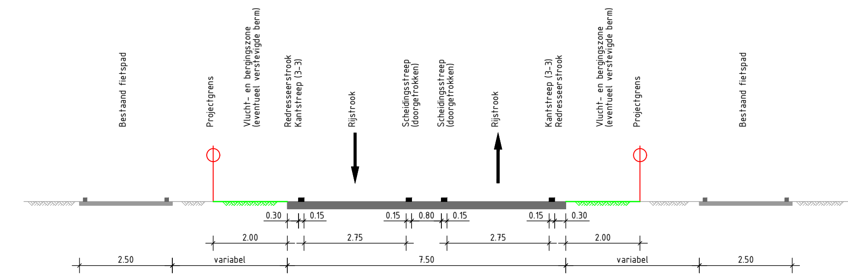
Principe dwarsprofiel A-A N285 - wegweg: rijbaan Schaal 1:100
