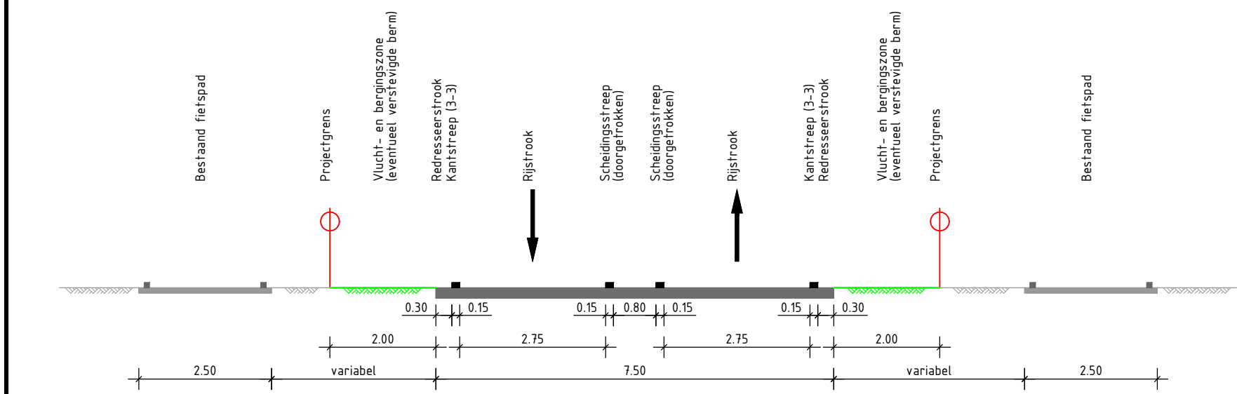
Principe dwarsprofiel A-A N285 - wegweg: rijbaan Schaal 1:100
