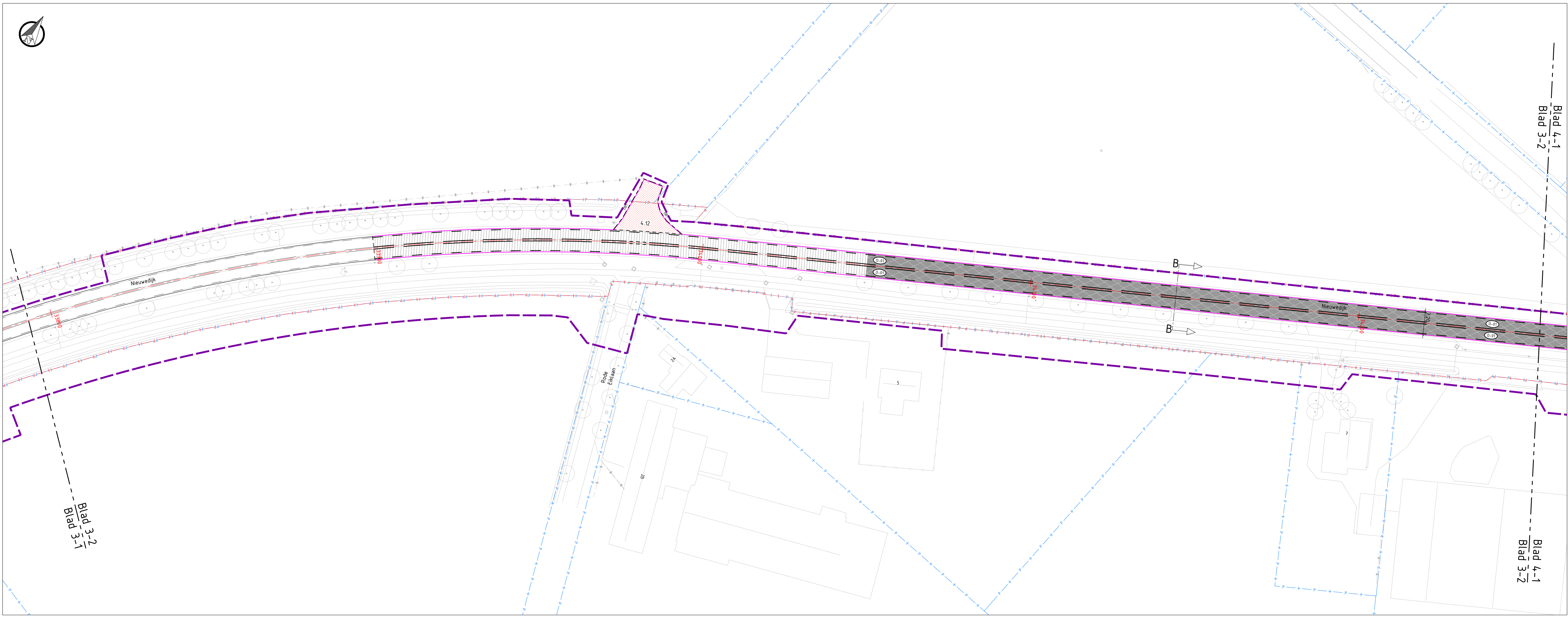
SITUATIE: BLAD 3-2 SCHAAAL 1 : 500
