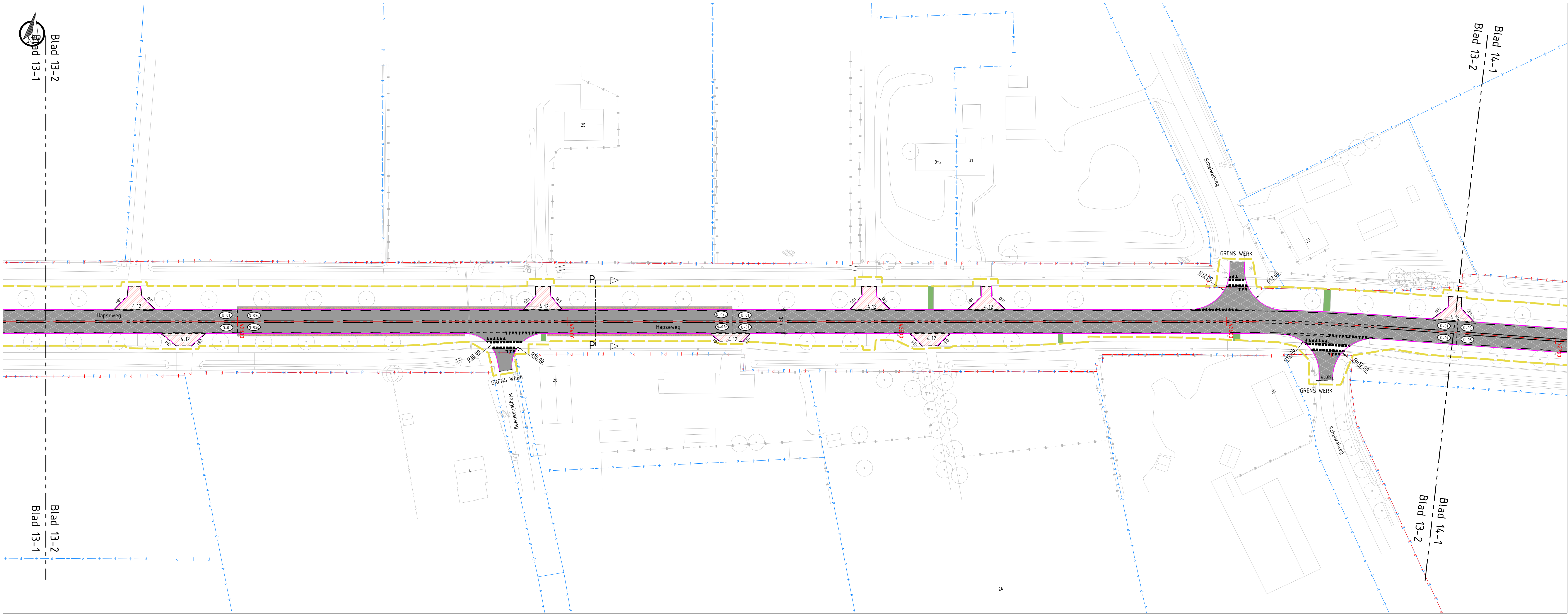
SITUATIE: BLAD 13-2 SCHAAL 1: 500
