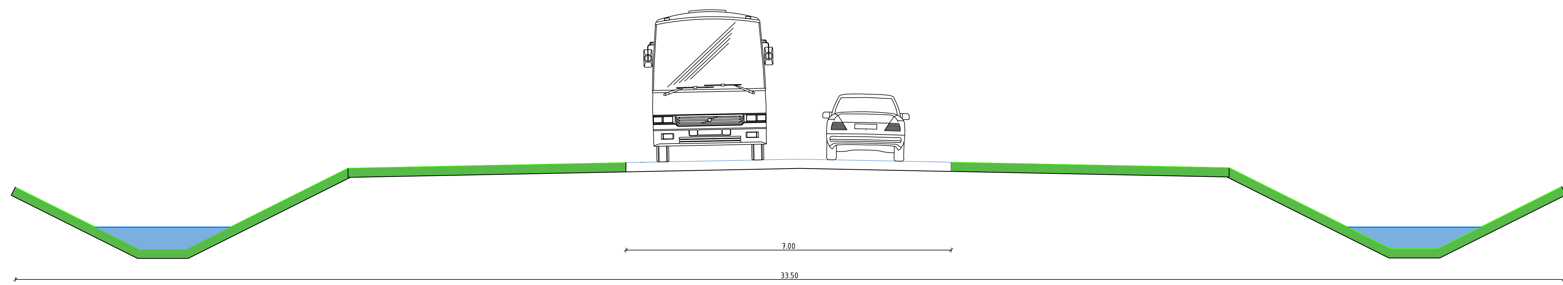
Dwarsprofiel onlegging Schaal 1:50
